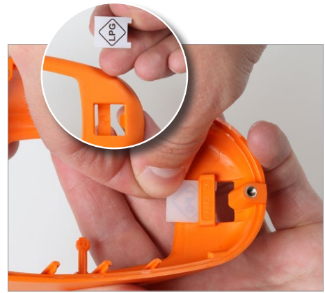
LPG-Kraftstoffkennzeichnung EK 867 FGI in Abdeckung oben EK 867 TSG einschieben. Attach LPG fuel grade identification EK 867 FGI to the top of scuffguard EK 867 TSG.
