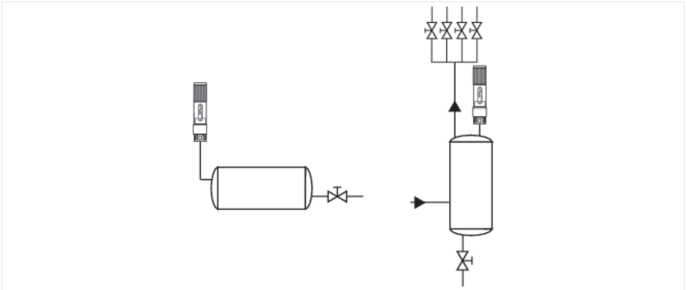
Abb. 1 Beispiel für den standardmäßigen Einbau des Sicherheitsventils
