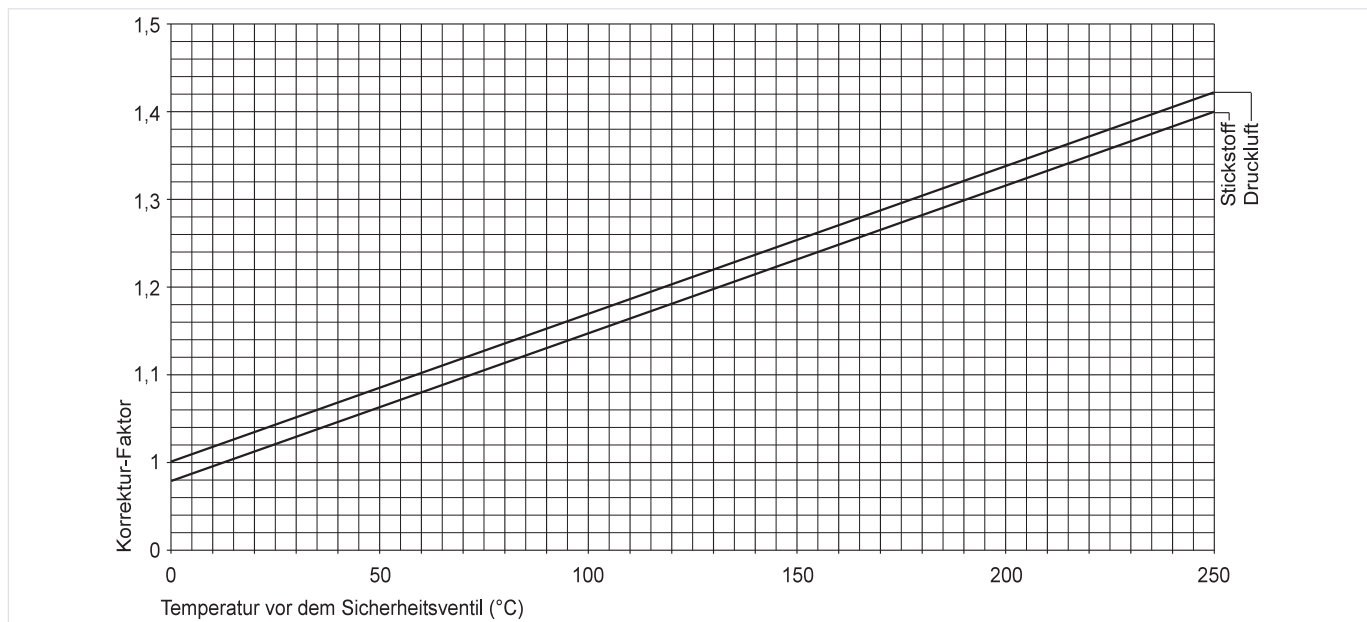
Abb. 2 Korrektur-Faktor in Abhängigkeit zur Temperatur
